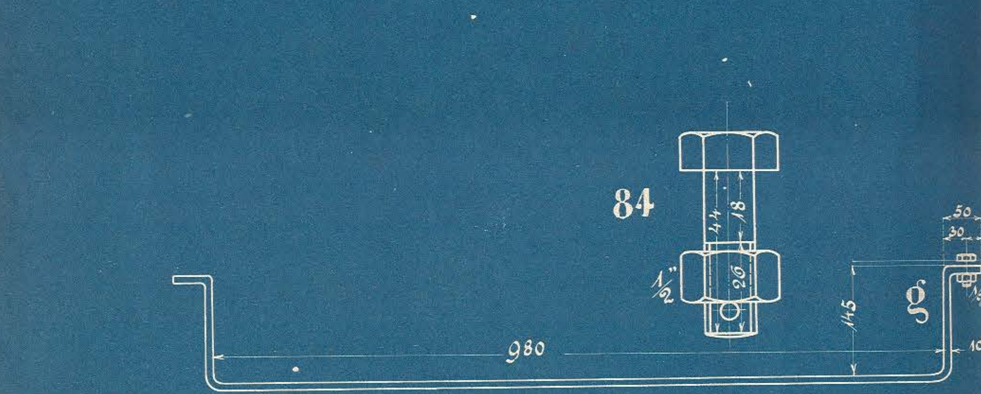
Bremsachse mit Lager u. Hebeln.
