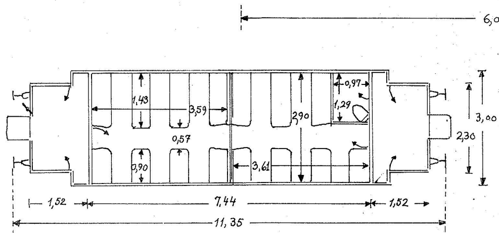
Indre indretning, skala 1:100 37 pl. III kl. På de fristående bænke er ryglænenene vendbare.
