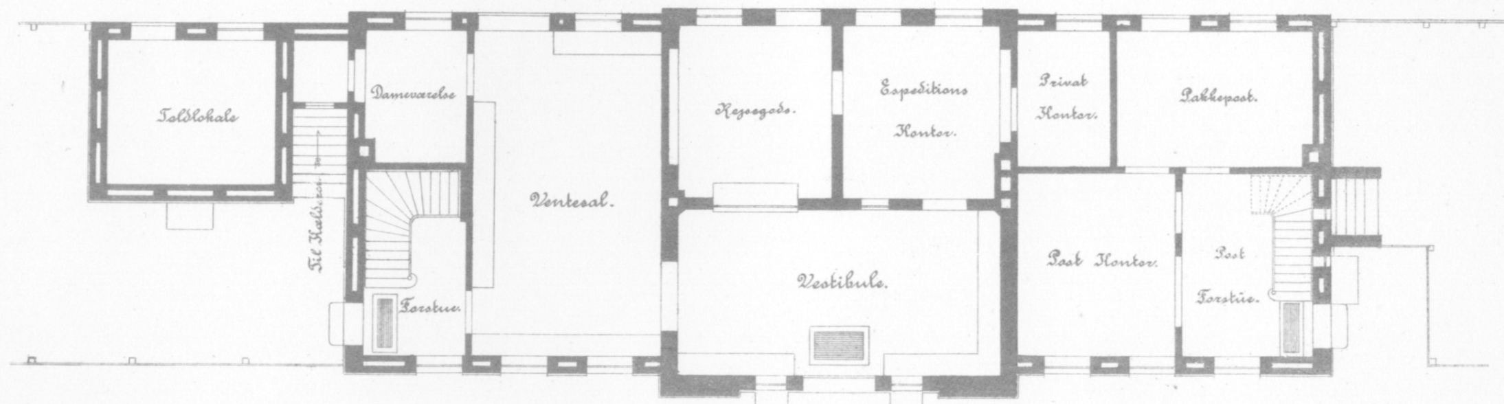
Plan af Stuen.
