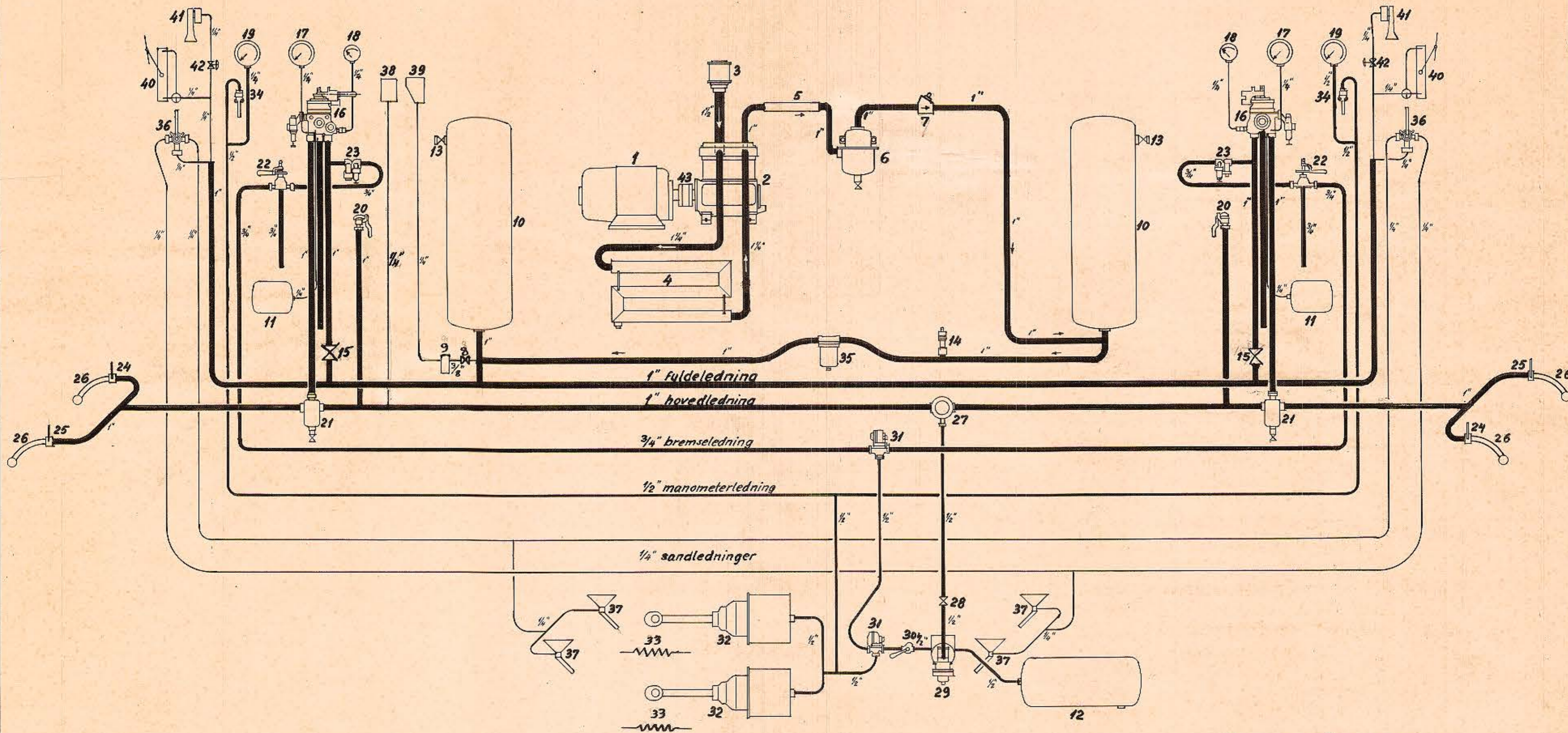
TRYKLUFT-RØRDIAGRAM ML 1208, 1209, 3202, 5203
