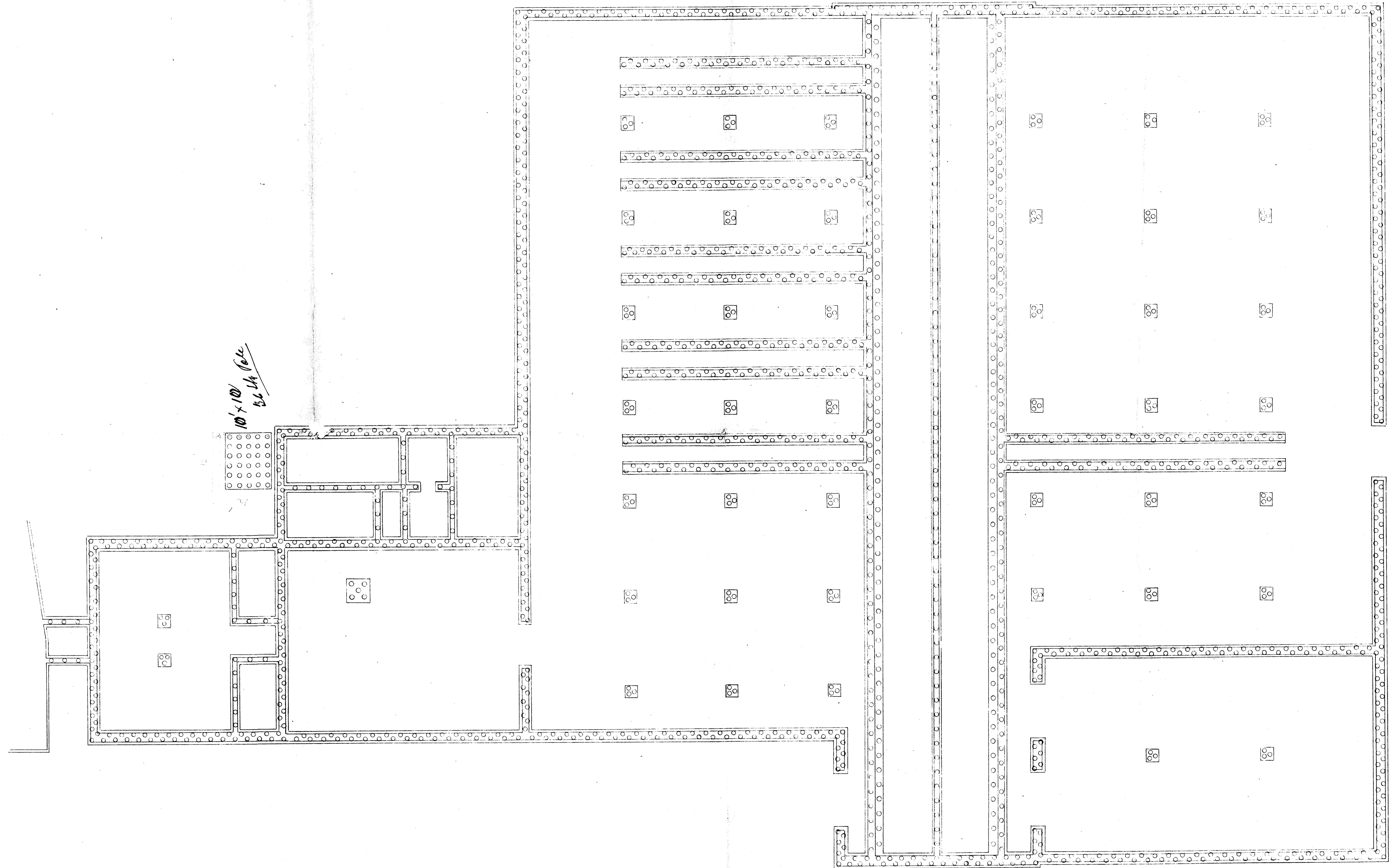
Plan af Bæsfundamentet.
