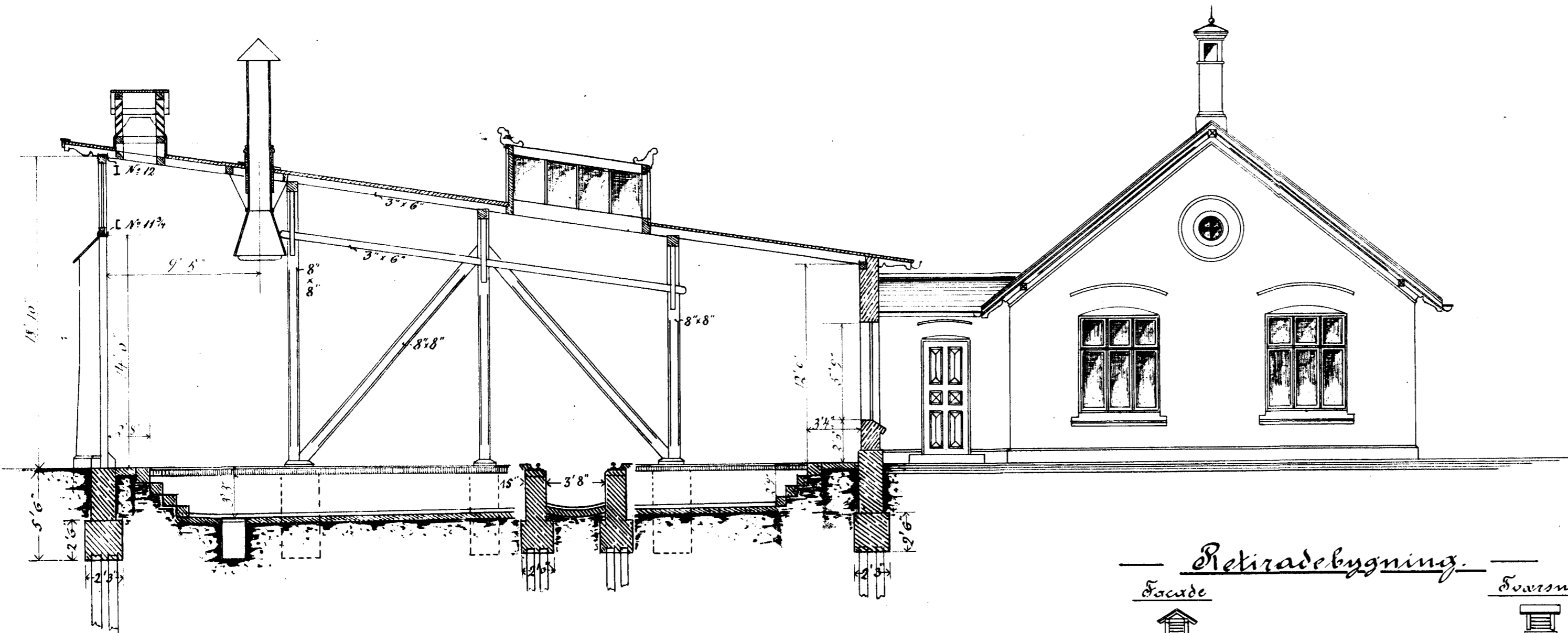
Gærfacade.
