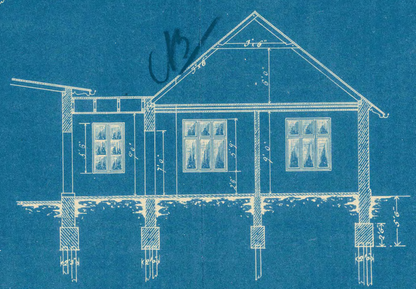
Snit e-d.
