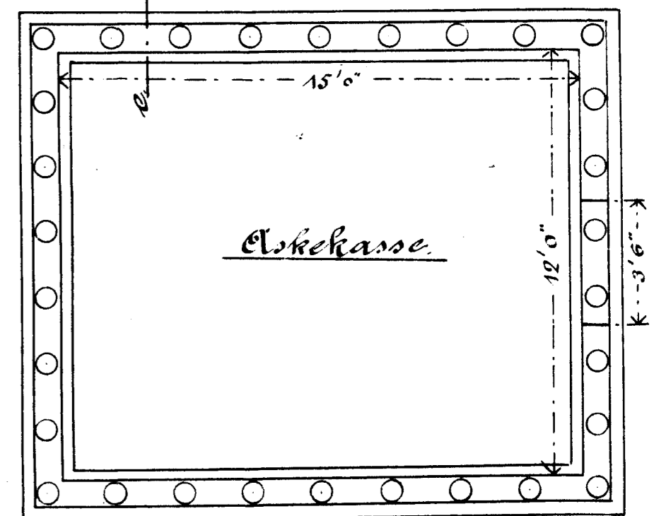
Snit e-d.
