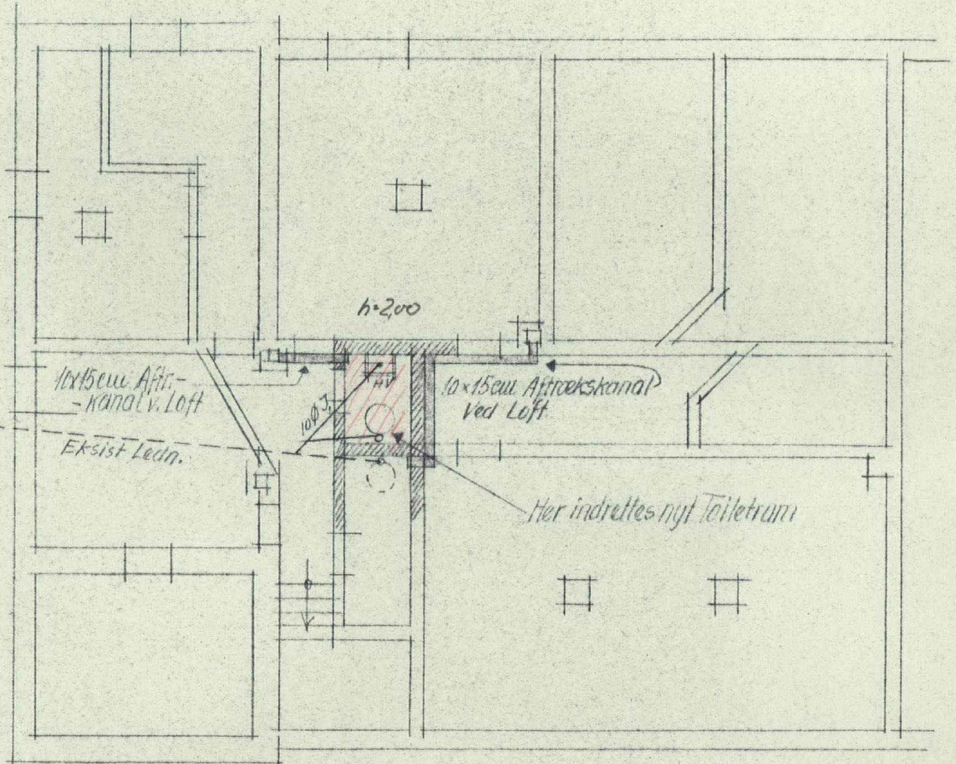
Kølderplan
