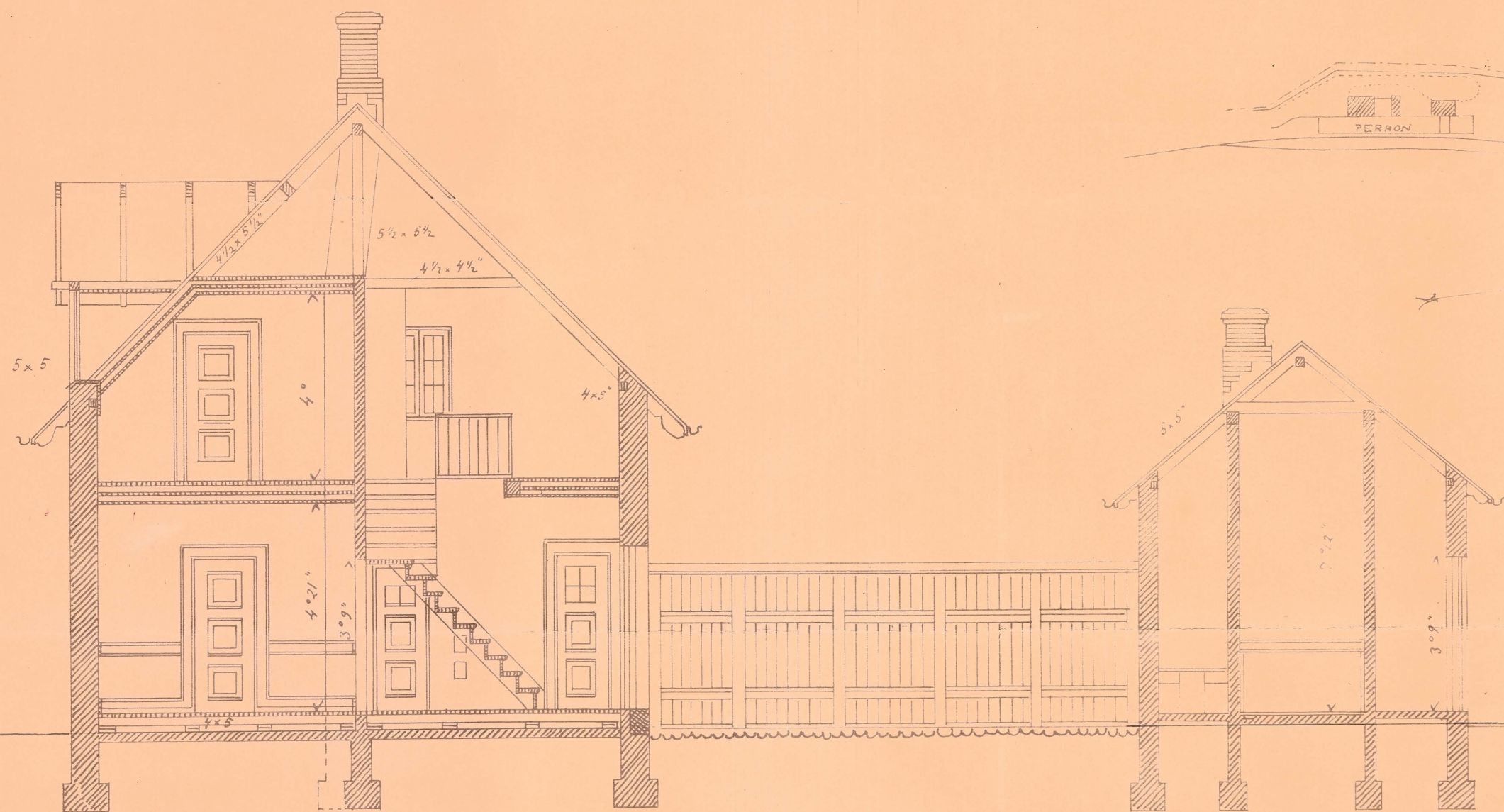
SNIT A-B
