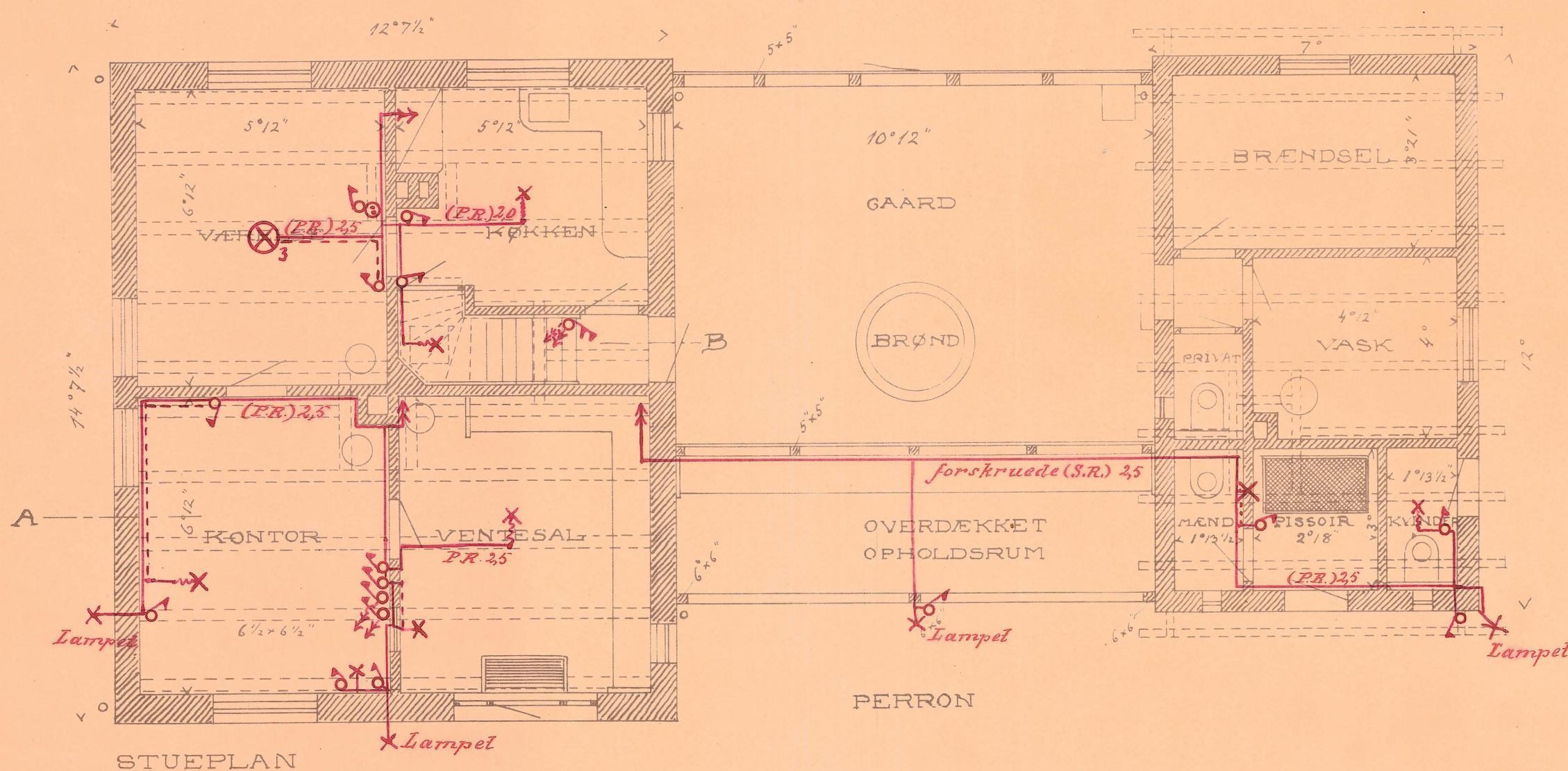
STUEPLAN
