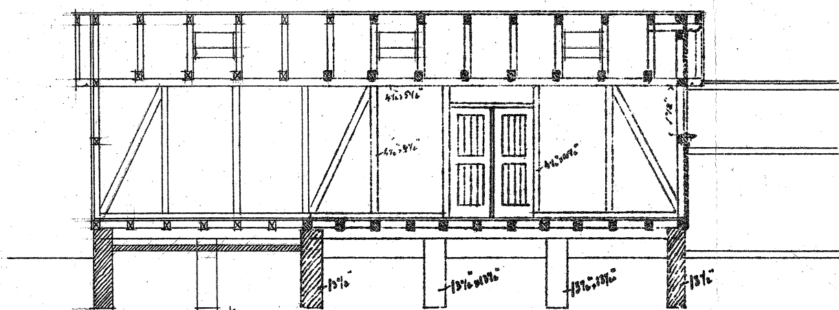
Snit B-B
