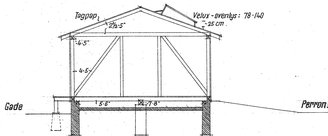
Snit A-A.
