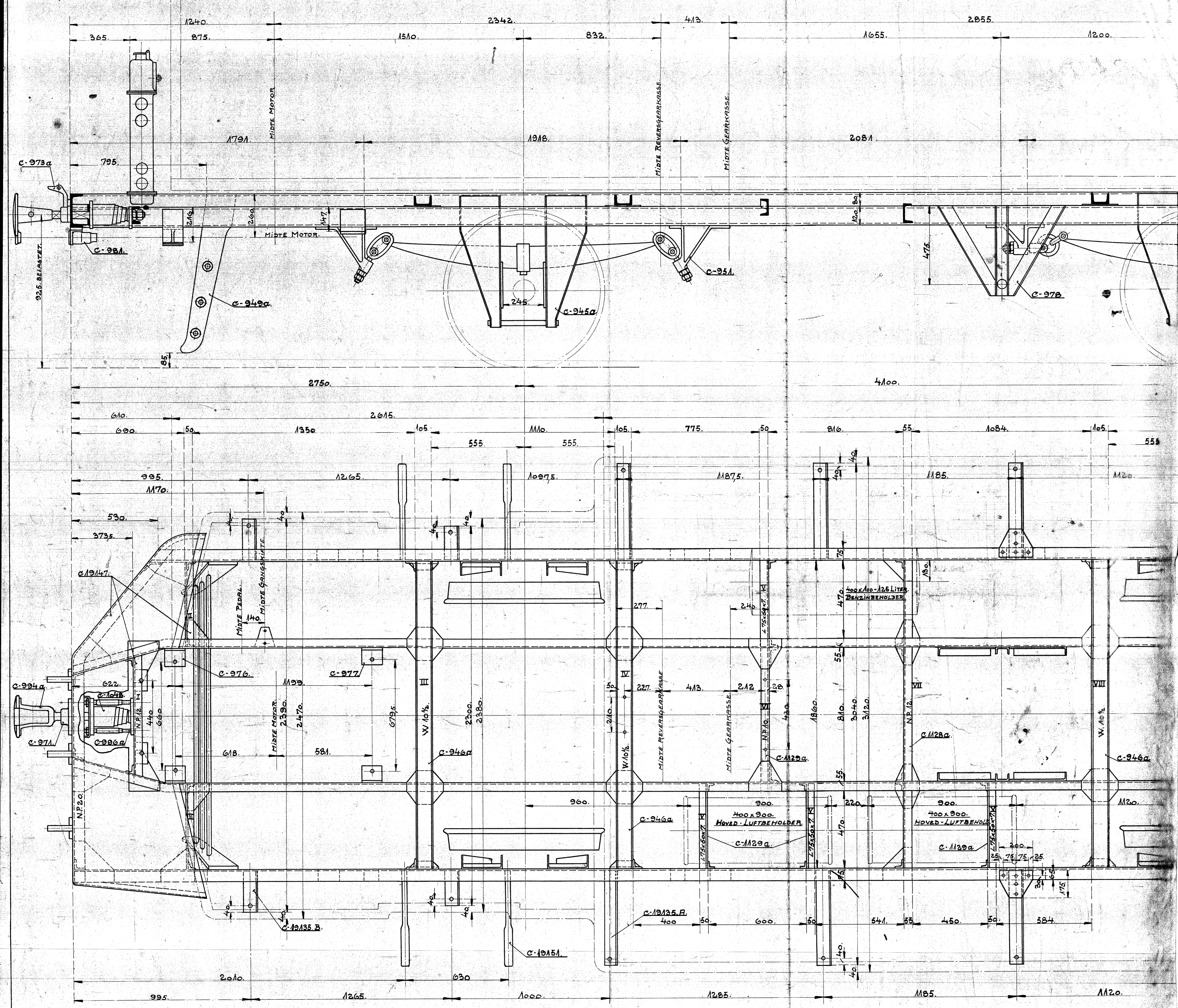
MONTAGETEGNING FOR MOTORVOGN. MODEL VI. SKALA 1:10.
