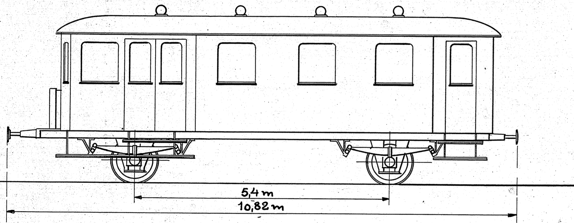
MOTORVOGN MODEL VII MED BAGAGERUM 42 SIDDEPLADSER
