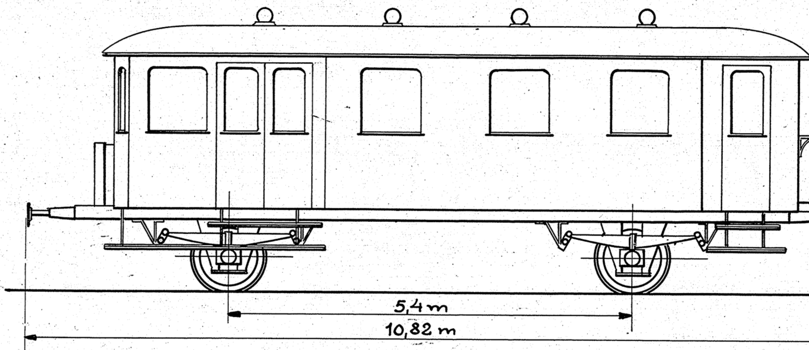
MOTORTOG MODEL VII 130 SIDDEPLADSER
