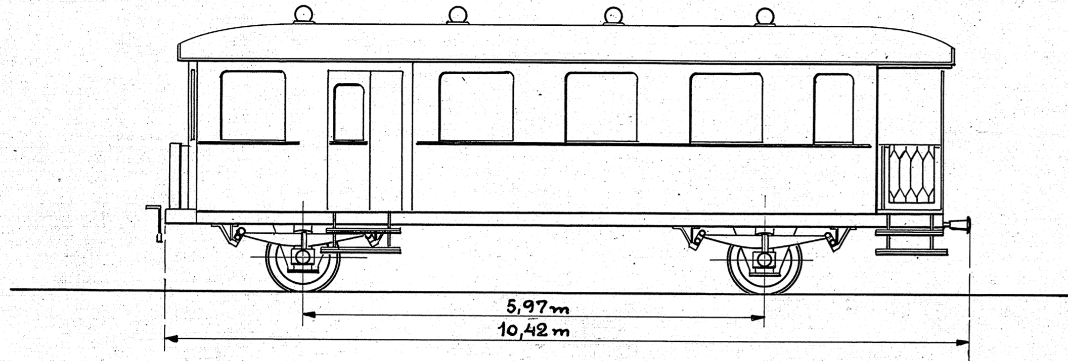
MOTORVOGN MODEL VII MED BAGAGERUM 42 SIDDEPLADSER
