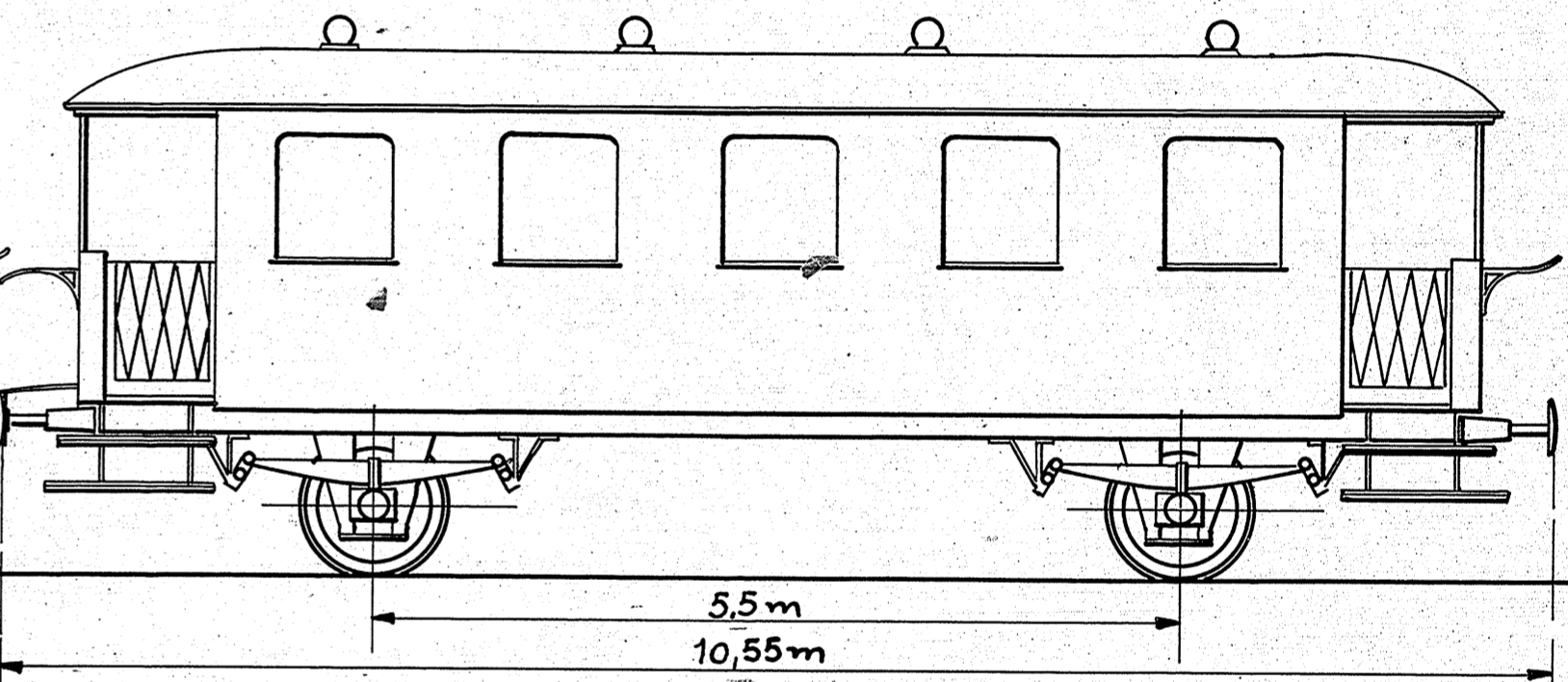
PAHÆNGSVOGN MED TOILETRUM OG AABNE PERRONNER 46 SIDDEPLADSER
