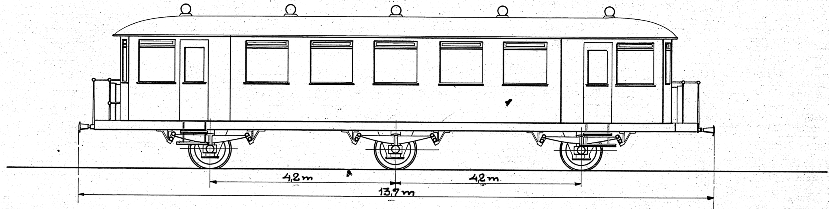
MOTORVOGN MED BAGAGERUM 42 SIDDEPLADSER
