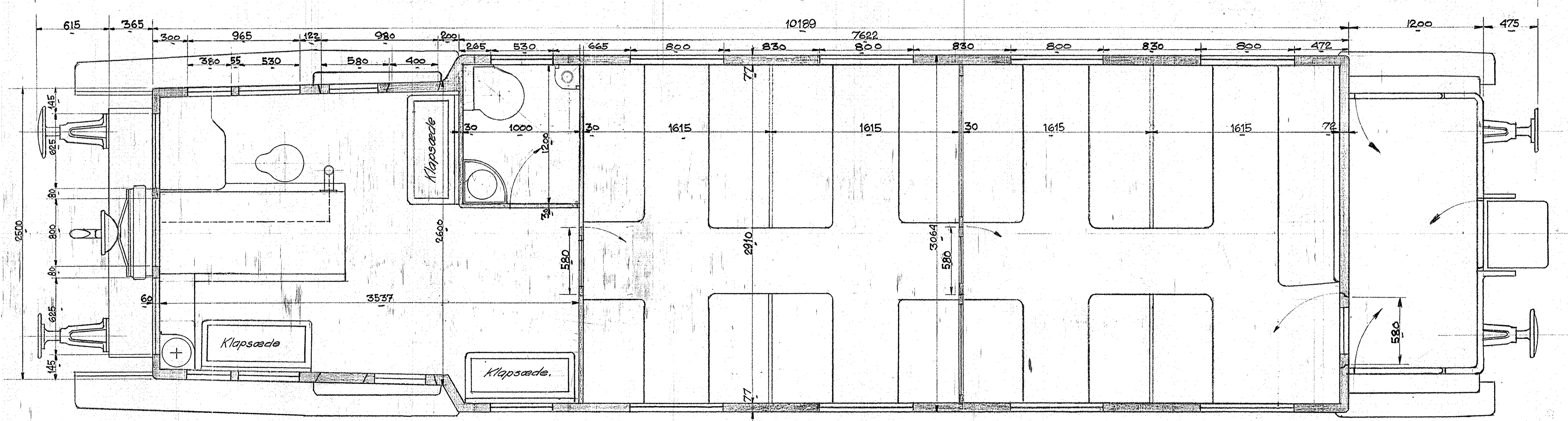
Ombygning af Personvogn til Motorvogn. 45 Siddepladser. Skala 1:20.
