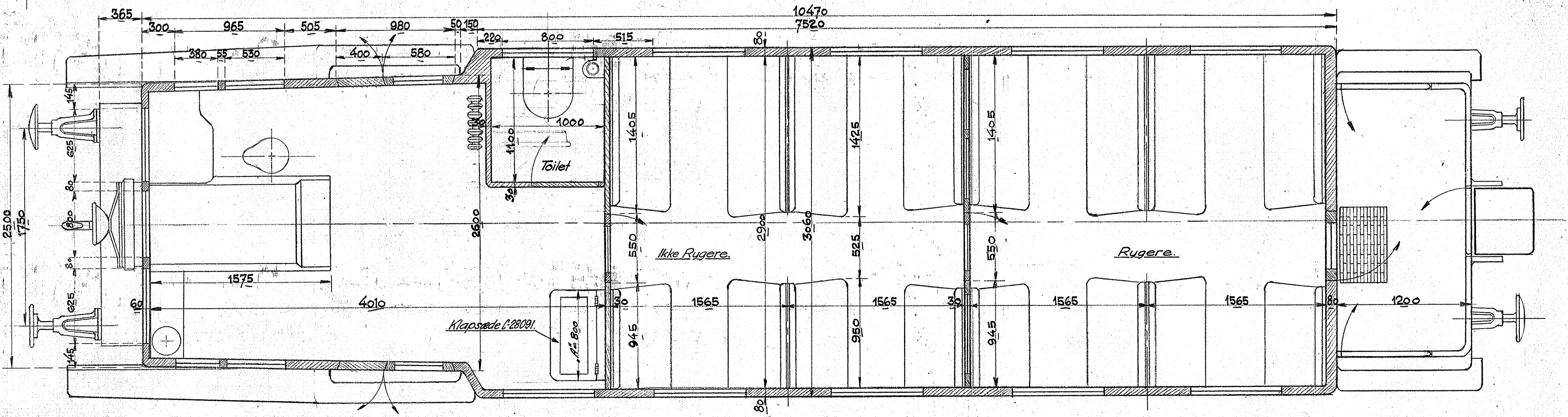
Ombygning af Personvogn til Motorvogn. - 42 Siddepladser.
