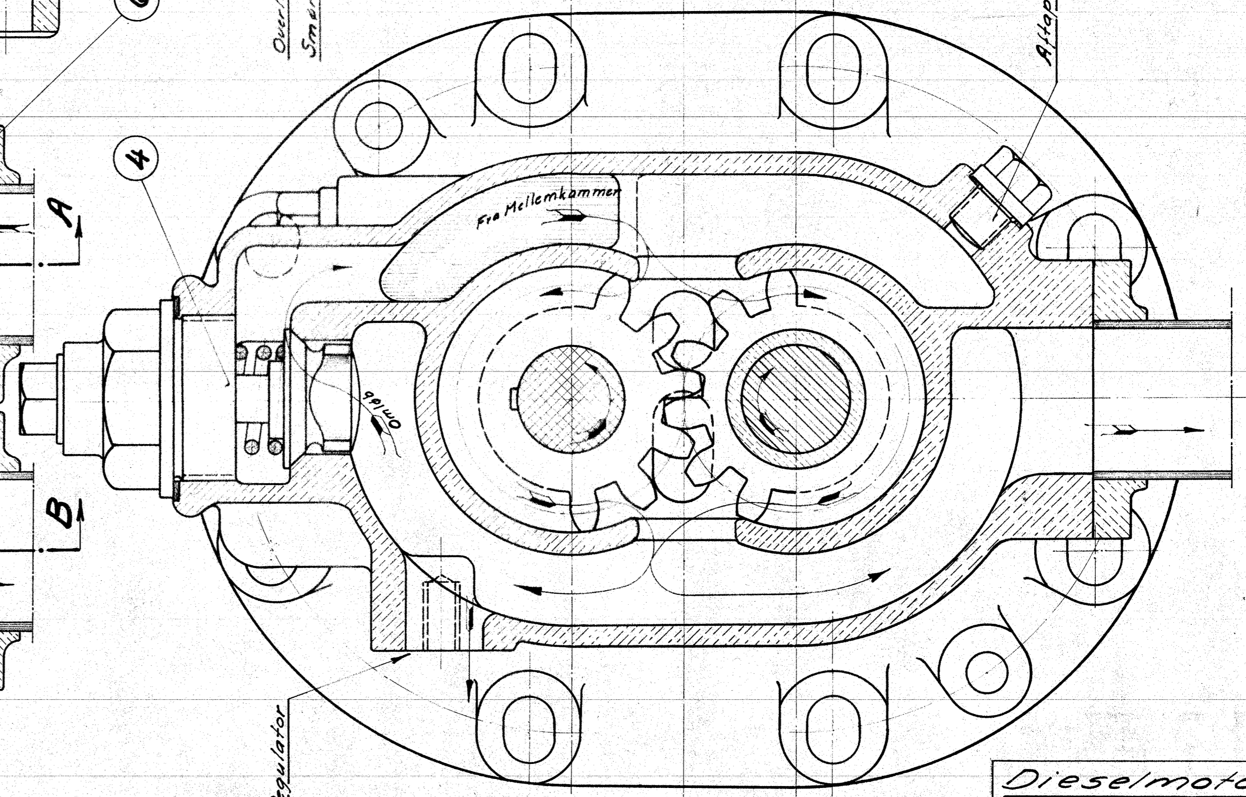
Snit B-B 2. Trin.
