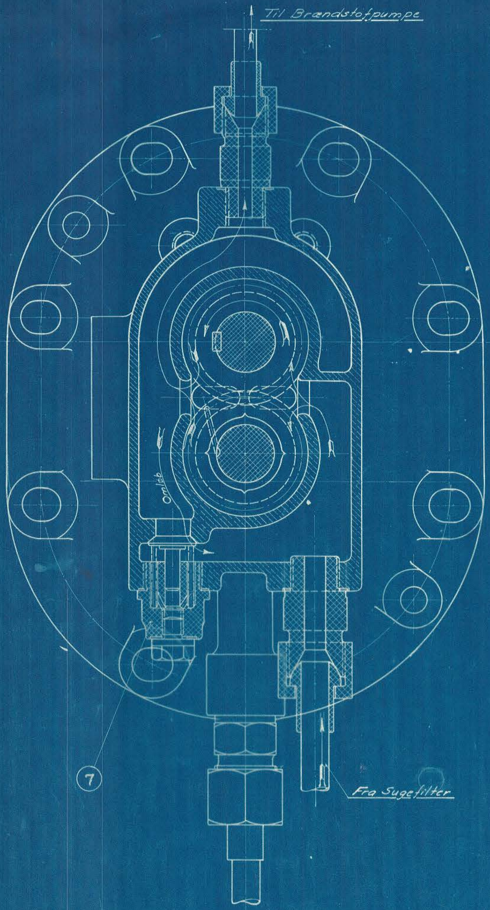
Snit A-A.
