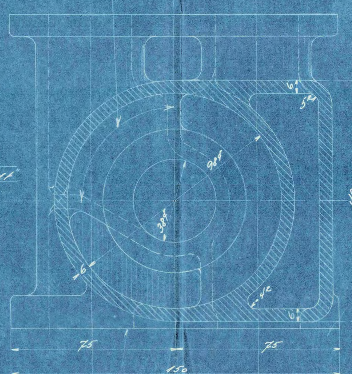
Snit D-D
