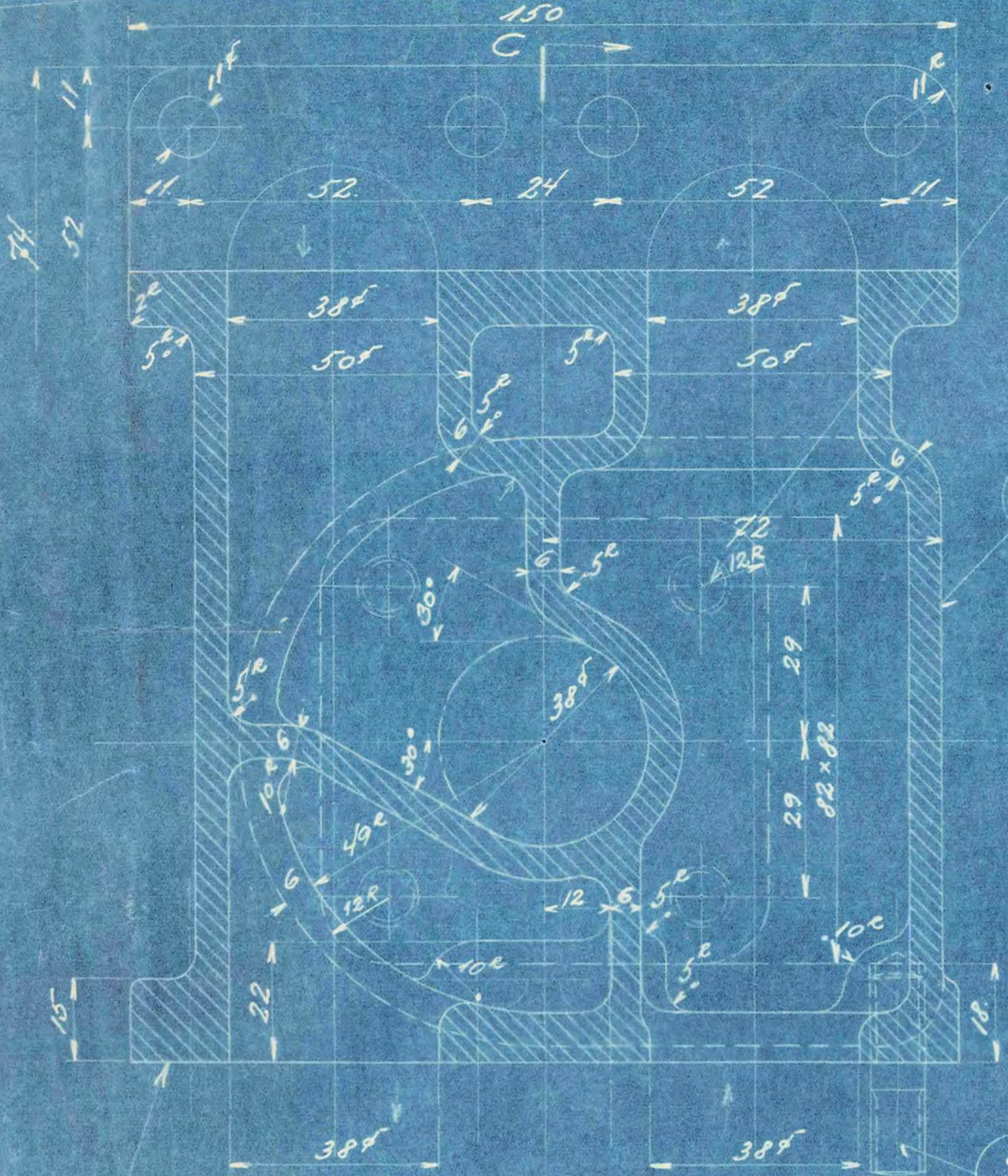
Snit B-B
