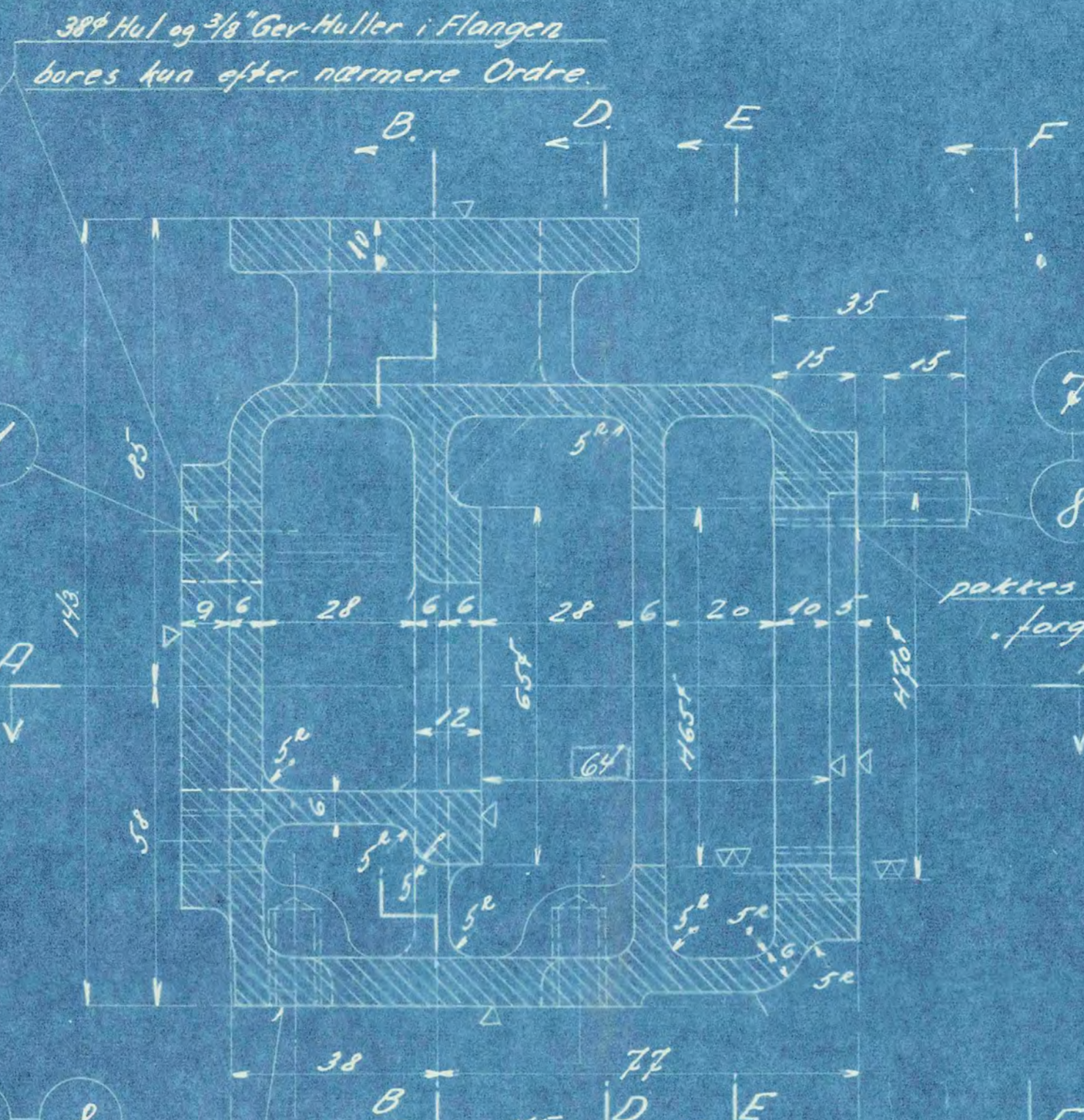
Snit C-C
