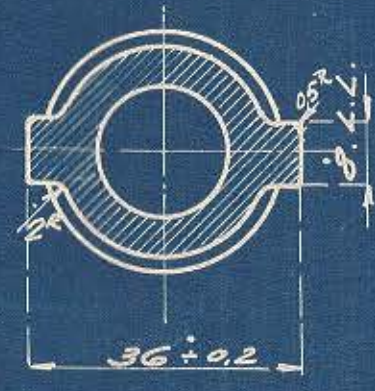
Snit A-A.
