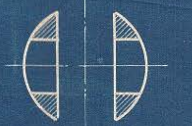
Snit B-B.
