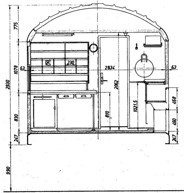
Snit B-B.
