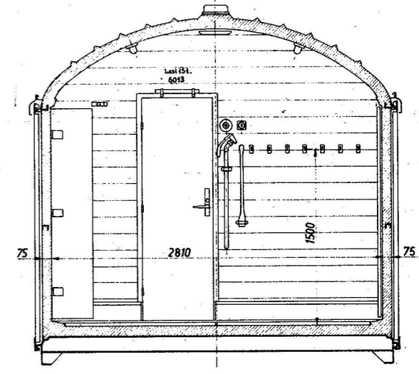
Snit A-A.
