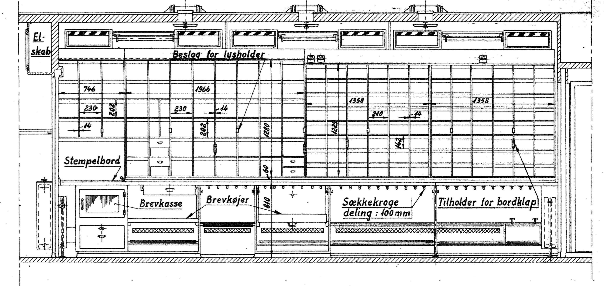
Snit G-G
