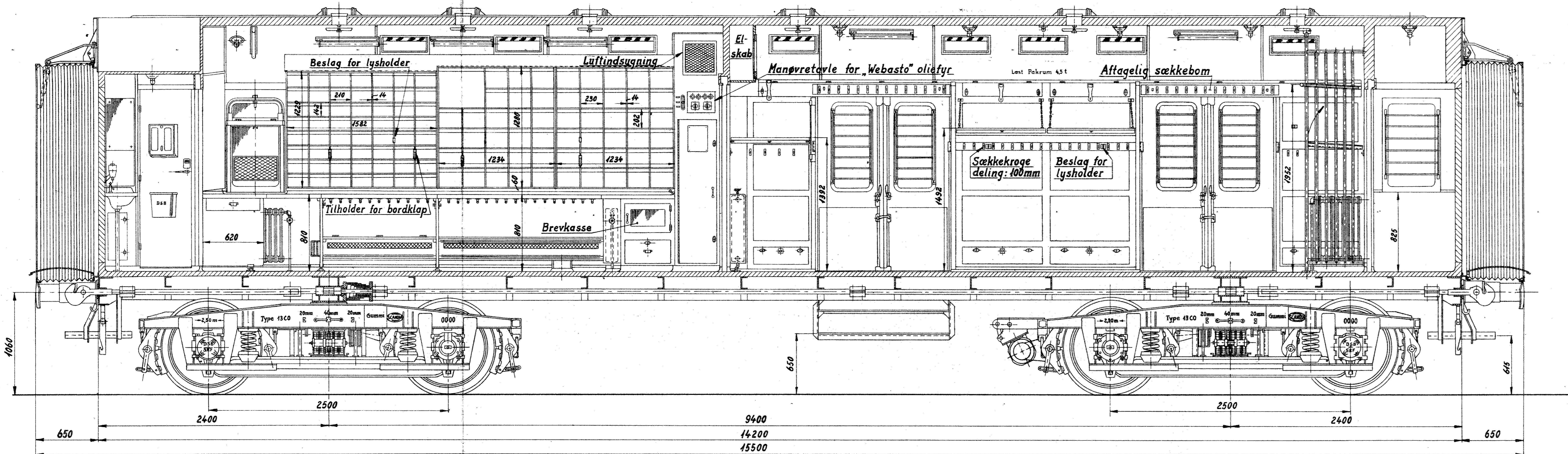
Snit A-A
