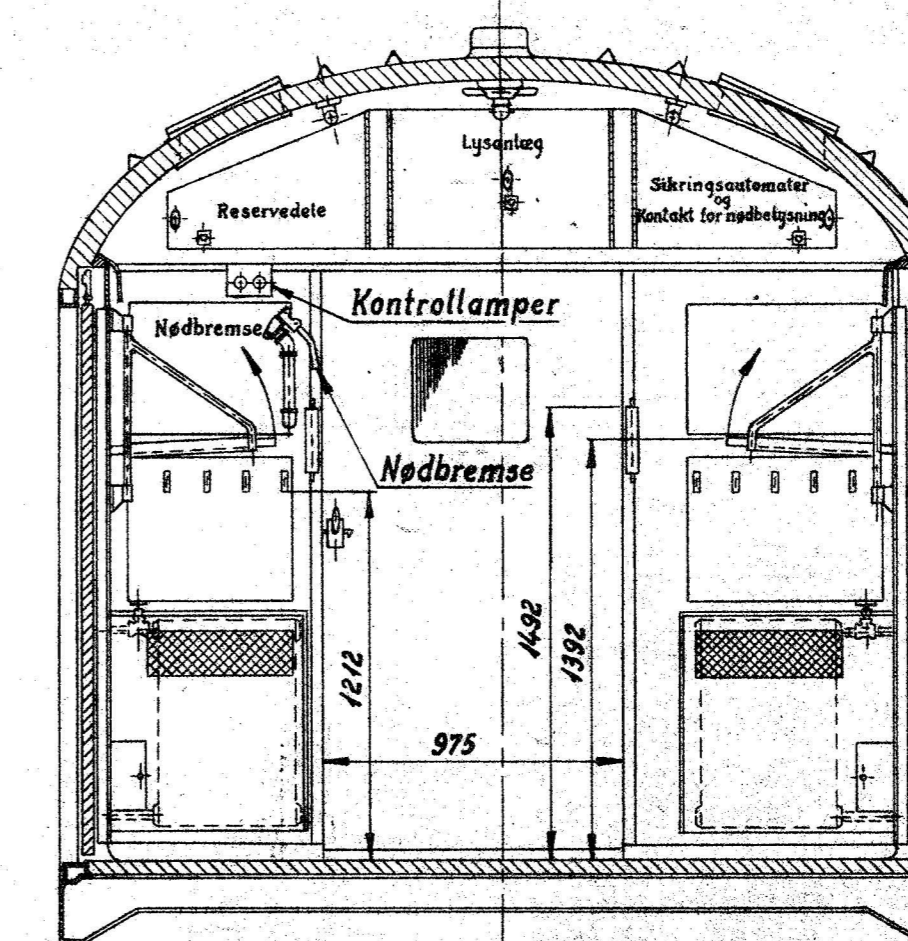
Snit E-E
