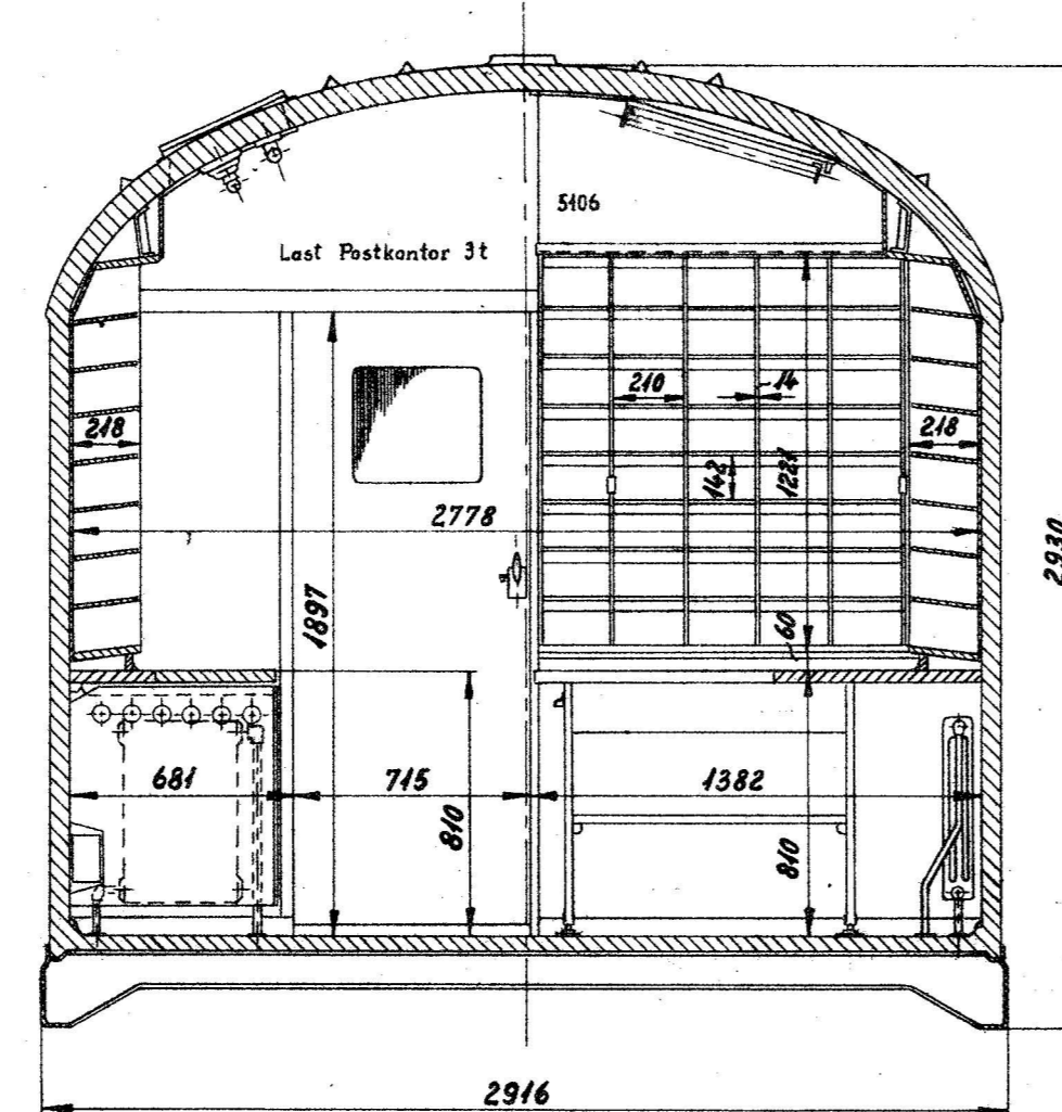
Snit C-C
