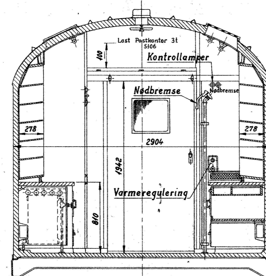
Snit D-D
