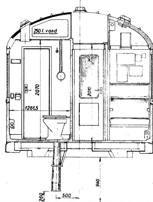
Snit d-d
