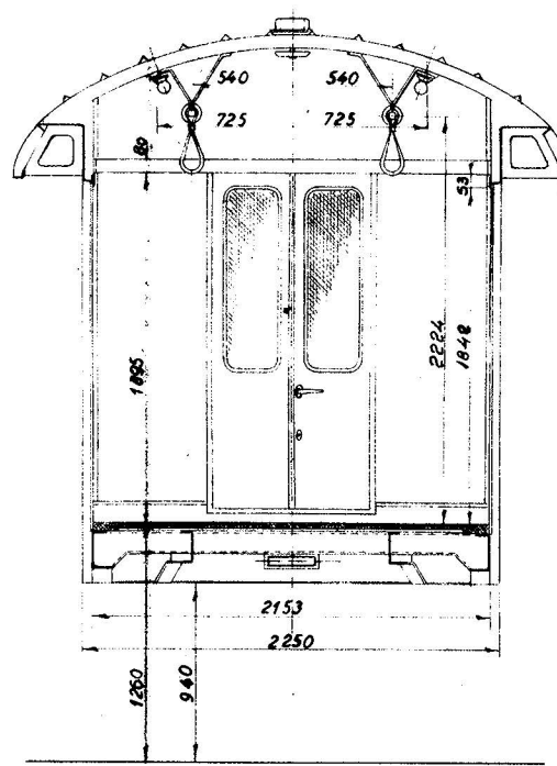
Snit b-b
