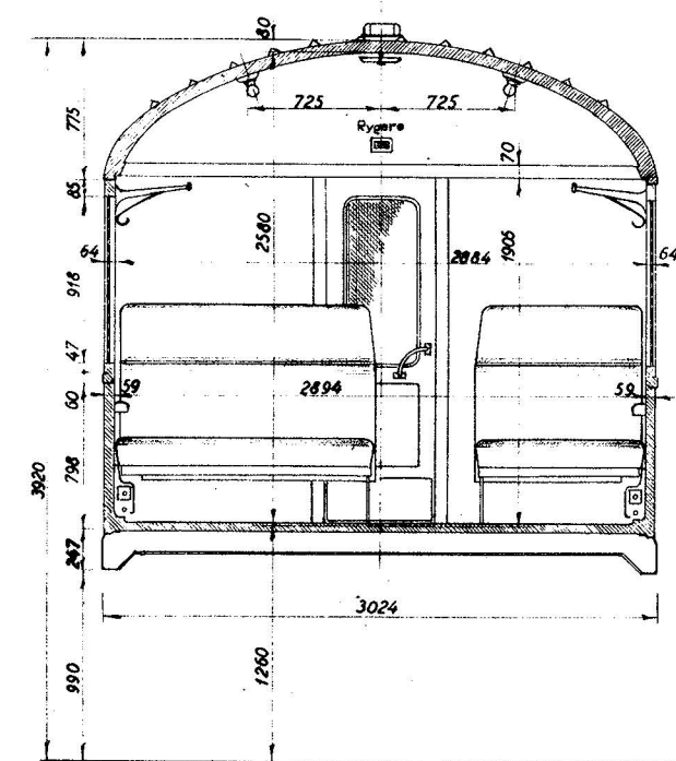
Snit c-c
