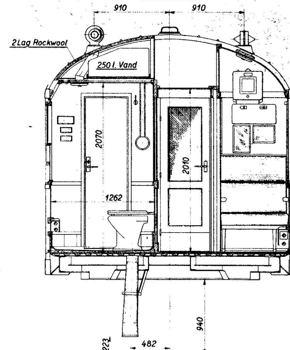
Snit-D-D
