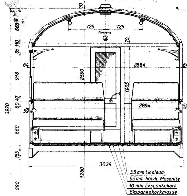
Snit-C-C
