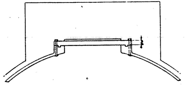
Detail af mandehul, 1:10
