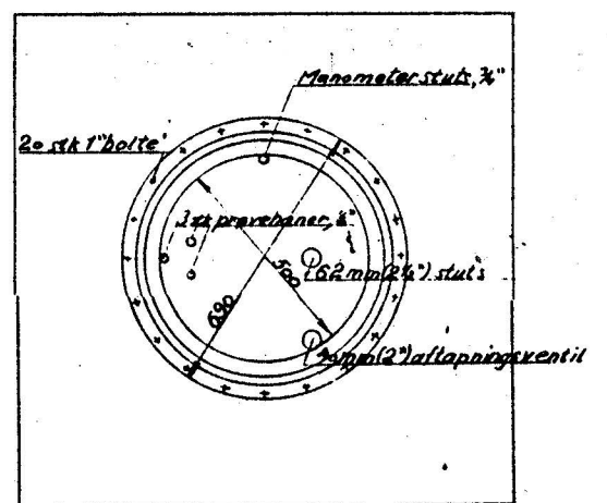
Detail af mandehul, 1:10
