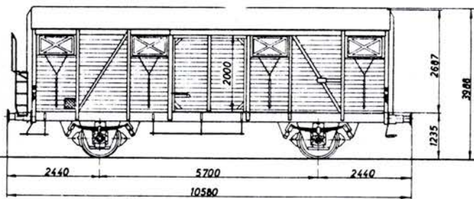
Lukket standardgodsvogn · Gs
