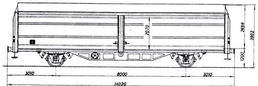
Lukket godsvogn med forskydelige sidevægge · Hbis
