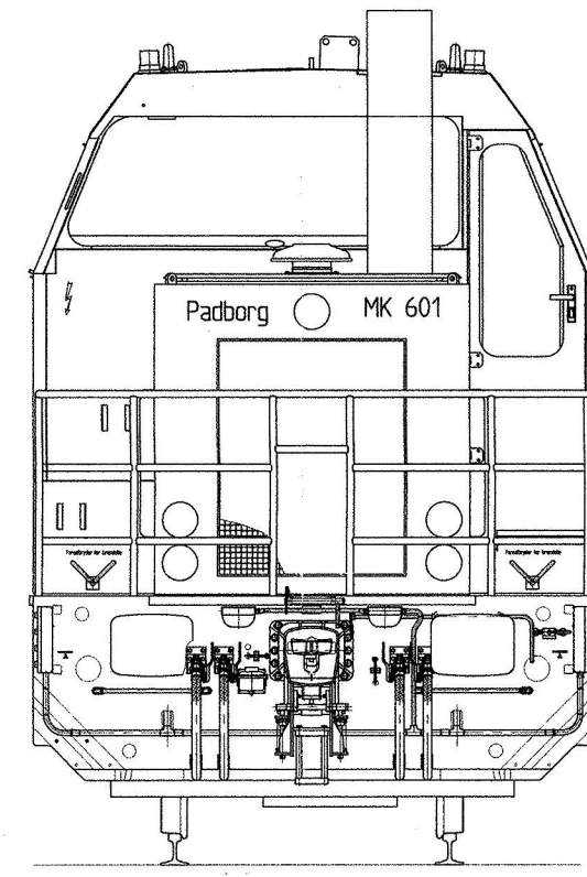
Vorderansicht
