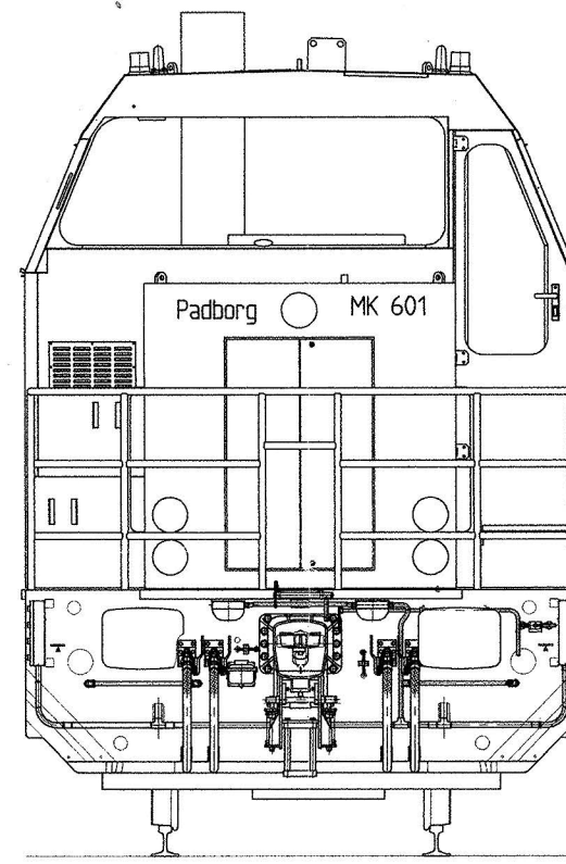
Rückansicht
