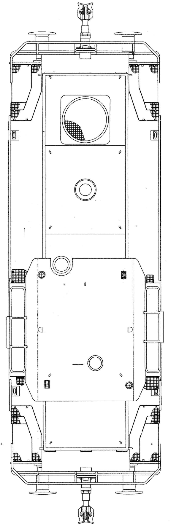
Draufsicht
