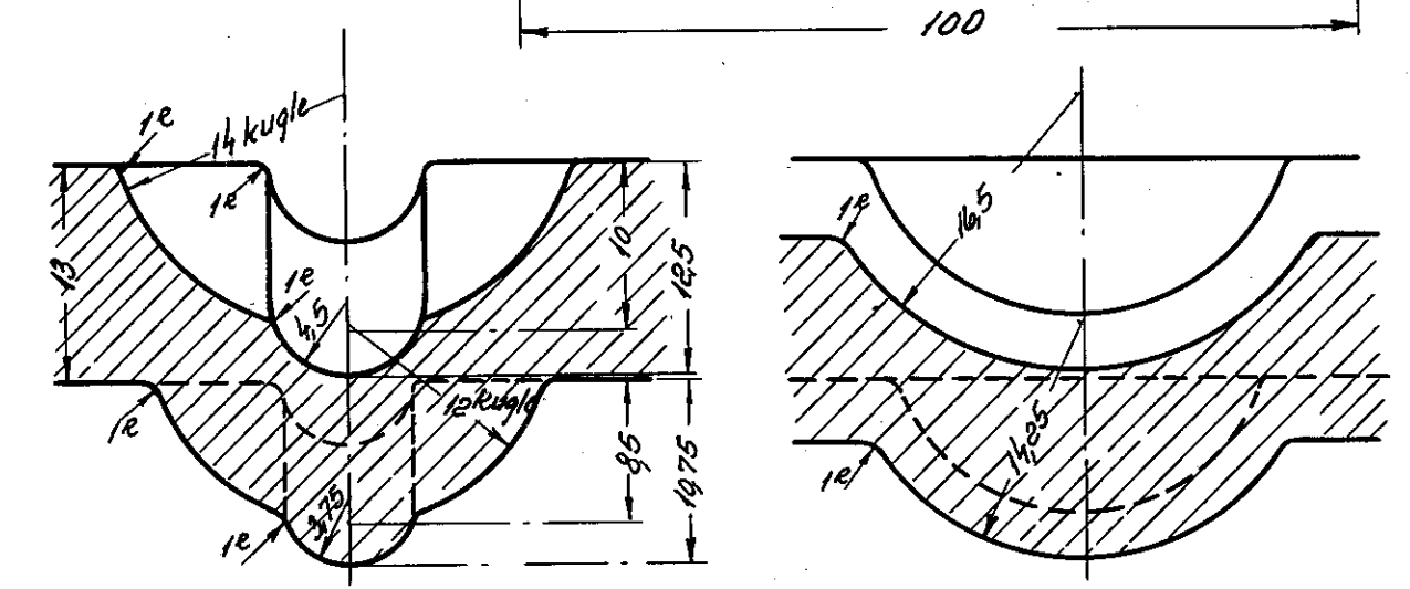
Tvoersnit: DIN 1571 2:1 Længdesnit.
